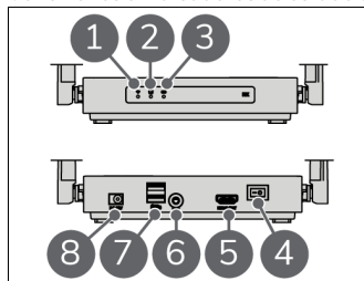
Figura 3: Receptor HDMI.
