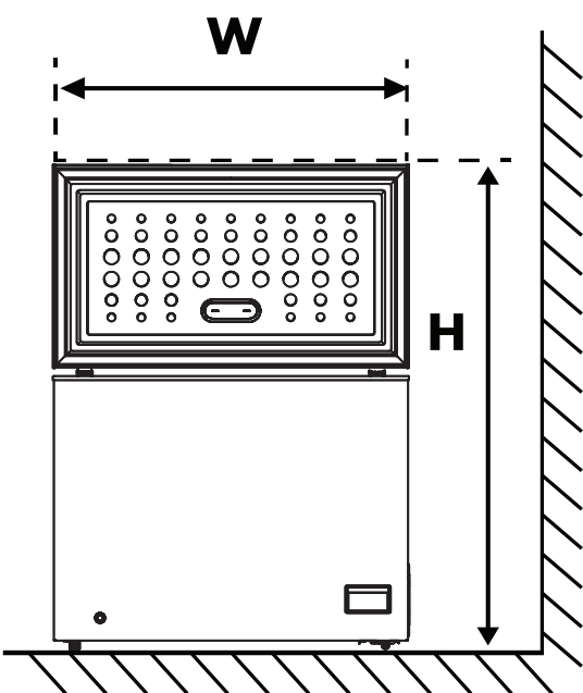
• Abbildung 1. Vorderansicht
